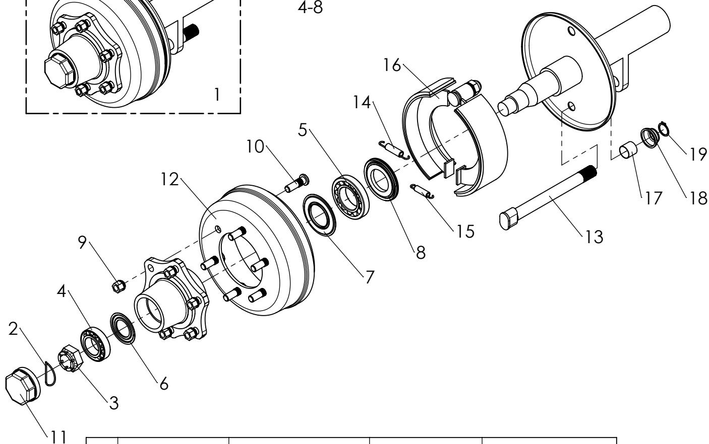
Laakerisarja/ Bearing kit V071LAASRJTVZ osat /parts: 4-8
